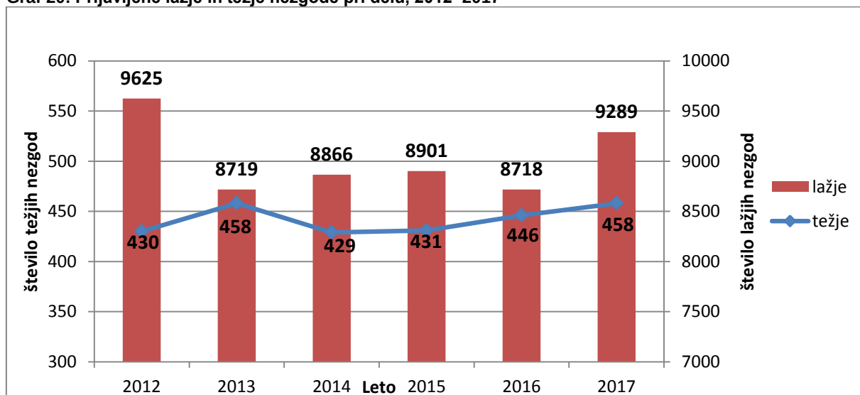
Graf 20: Prijavljene lažje in težje nezgode pri delu, 2012–2017
